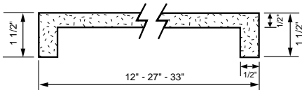
Bar Top CFB-120, CFB-270, CFB-330
